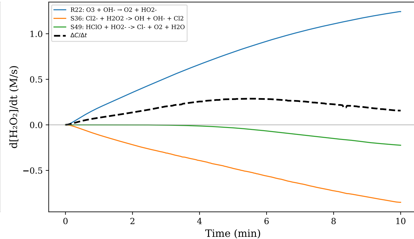
(d) \text{H}_2\text{O}_2
